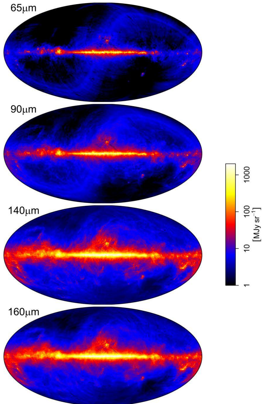
図2 : 「あかり」は4つの波長で遠赤外線全天画像を作成した。図の上から順に 65 マイクロメートル、90 マイクロメートル、140 マイクロメートル、160 マイクロメートルの各全天画像を示す。中央に水平に伸びる天の川が各画像で明るく見える。一方、波長の長い画像は、より低温の星間物質の分布を示し、このような物質は天の川から上下方向により広がっていることが分かる。この差は 90 マイクロメートルと 140 マイクロメートルの 2 波長の画像の間で特に顕著である。100 マイクロメートルより短波長の 2 画像がこれまで「IRAS」により観測されていた遠赤外線の描像、一方 100 マイクロメートルより長波長の 2 画像が「あかり」が新しく描き出した遠赤外線の全天の詳細な分布である。
