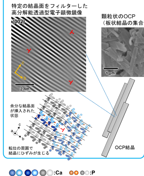
図 高密度で転位を導入したリン酸八カルシウム(OCP)が発現する高い自己溶解性に伴う新生骨置換性の説明と概要(⊥で示された位置の刃状転位の転位線は、紙面と直交する)。
