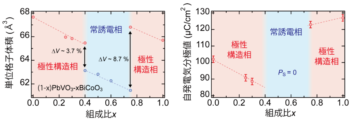
図 2 : (1-x)PbVO 3 -xBiCoO 3 固溶体における単位格子体積と自発電気分極の変化 (室温)
