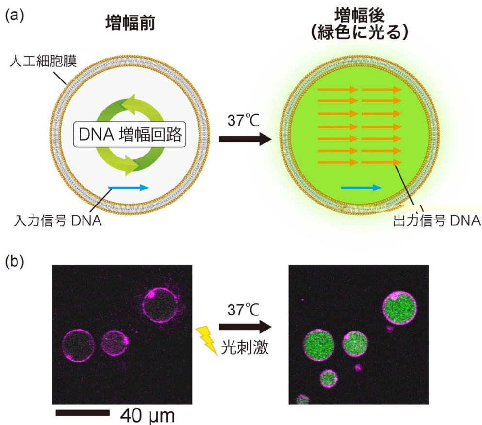
図 2: (a) DNA を増幅する人工細胞の模式図. 人工細胞膜の中に DNA 増幅回路が封入されている. 入力信号 DNA に応じて回路が動作し, 37°C 下で出力信号 DNA を産出・増幅する. (b) 光刺激による DNA 増幅開始制御の様子を撮影した顕微鏡画像. 人工細胞膜はマゼンタ色で示されている.
