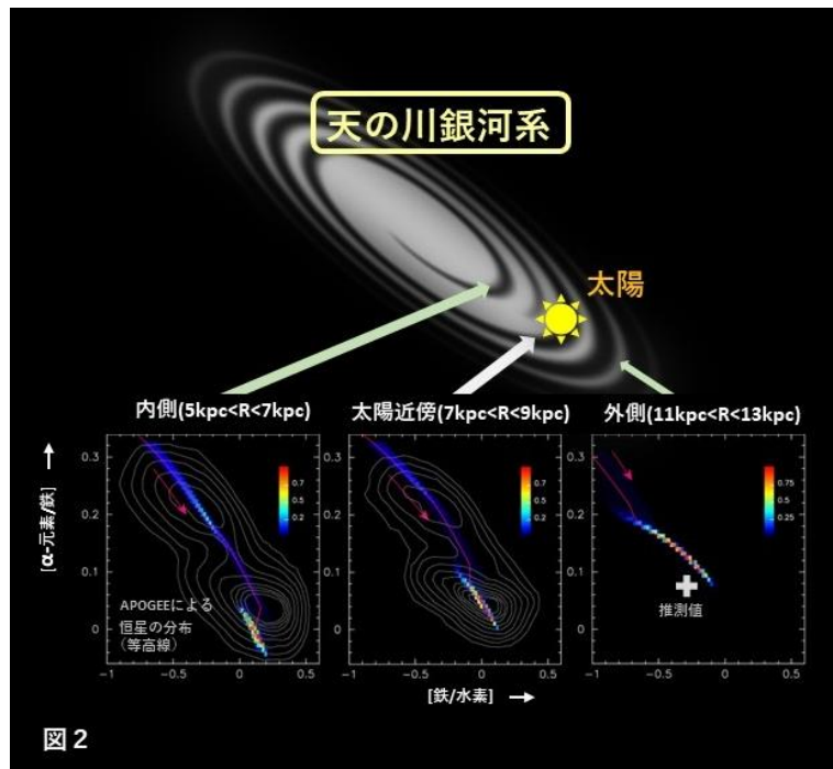
図2：天の川銀河の異なる場所における星の元素組成分布。中心からの距離 R によって天の川の円盤を3つの領域に分けた。太陽は中心から約8 kpcの距離にある。カラーマップは野口准教授のモデルを示す (Credit: M. Noguchi, Nature, July 26th 2018 issue)。等高線はAPOGEEによる内側と太陽付近における星の頻度分布を示す (Credit: M. Haywood et al. A&A, 589, 66 (2016), reproduced with permission © ESO)。中心に近いほど、 \alpha 元素の豊富な星の割合が増える様子がモデルでも再現されている。
