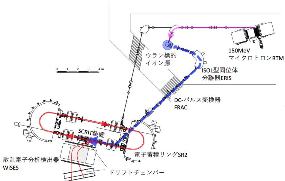
図 3 SCRIT 電子散乱実験施設（新型電子顕微鏡システム）
