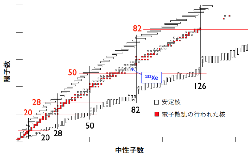
図1 電子散乱の行われた原子核を示した核図表
