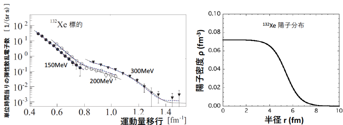
図6 弾性散乱の運動量移行分布（左）とそこから決められた 132 Xeの陽子分布（右）
