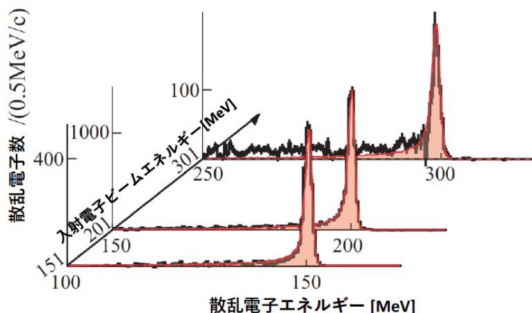
図5 散乱電子のエネルギー分布
