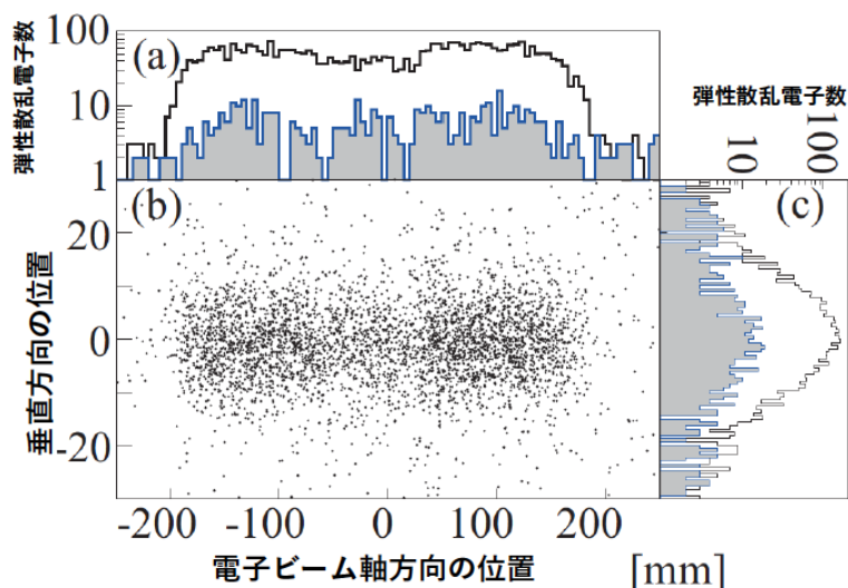
図 4 散乱地点の分布
